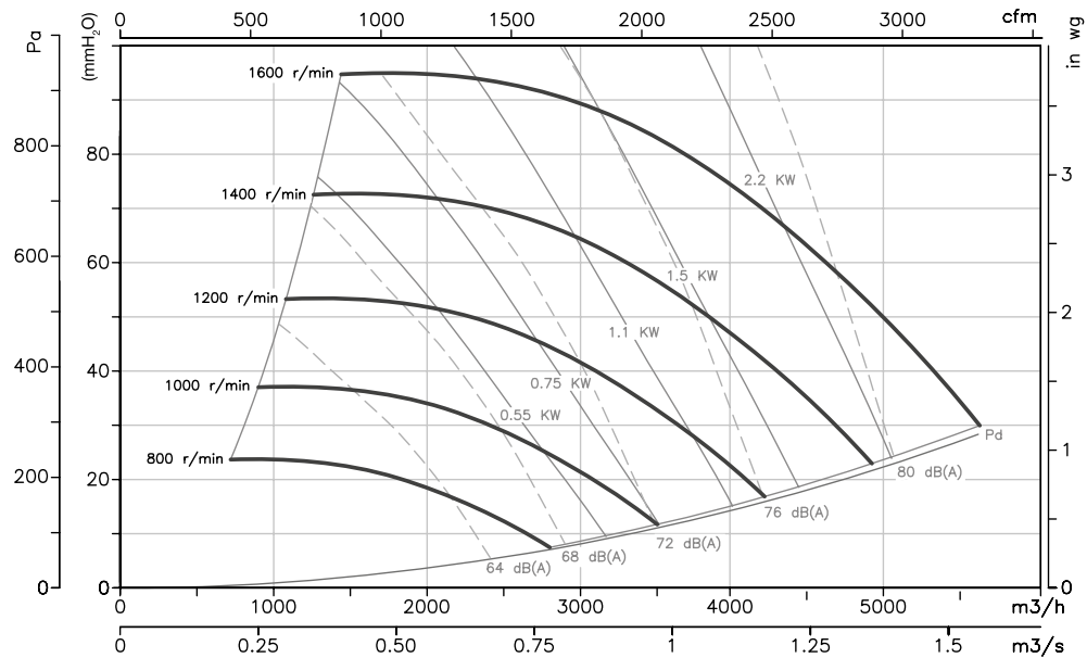
CJSX-12/6
