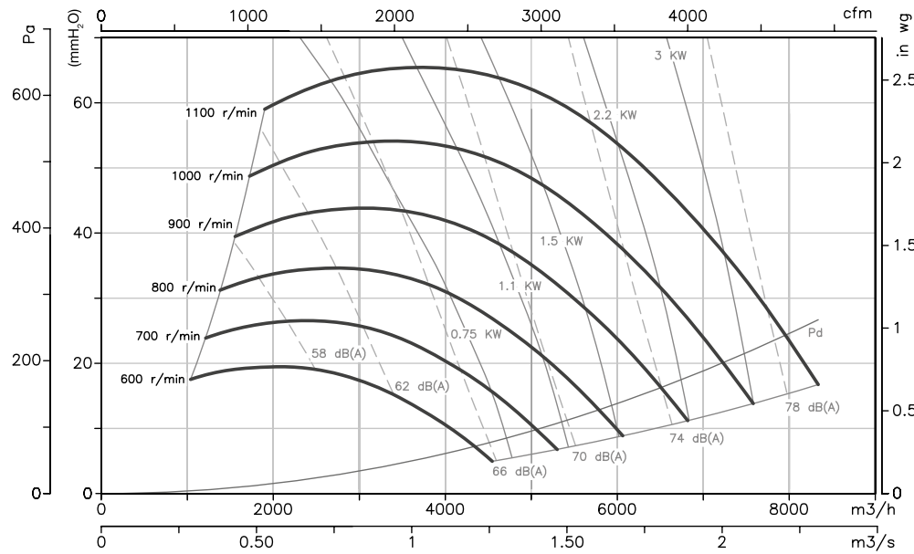
CJSX-15/7
