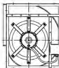
CBDT-18/18
